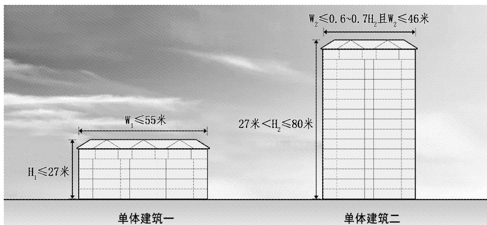
附录5 单体住宅建筑形体示意图
